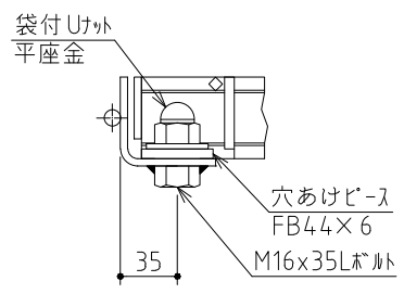
ボルト固定部詳細
