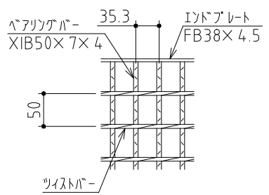
グレーチング構造図
